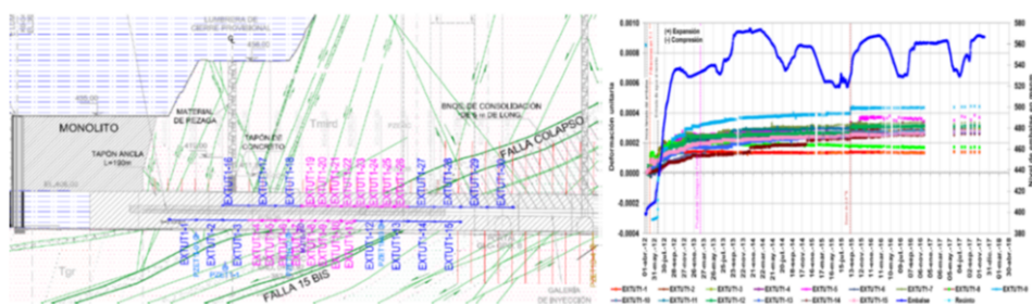
Figura 2. Instrumentación instalada en los túneles ancla o tapones estructurales de presa La Yesca. Figura cortesía de la CFE, GEIC.
