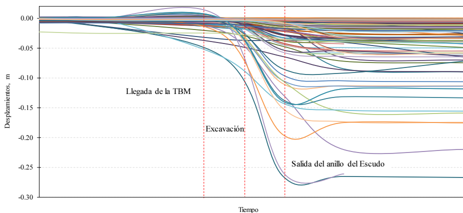
Figura 10. Conjunto de perfiles de asentamientos del intertramo.
